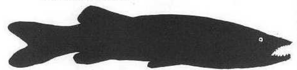
Pickarel Esox Lucius
