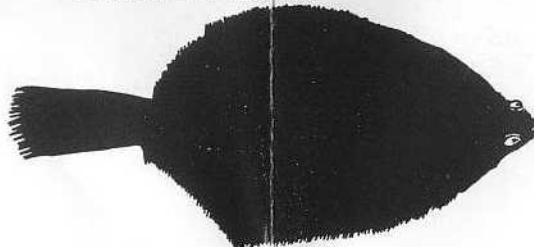
Dab Limanda Limanda
