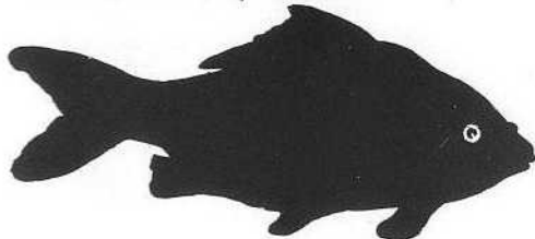
Chub Leusiscus Cephalus
