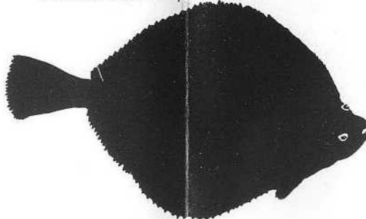
Plaice Pleuronectes platessa
