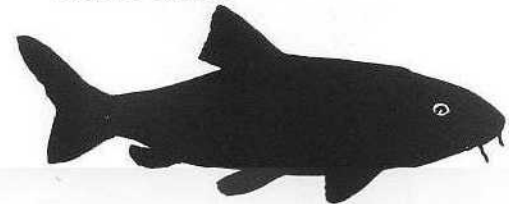
Barbel Barbus barbus
