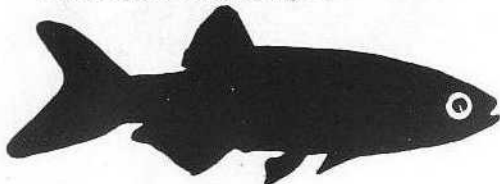
Danio Laubuca Dadiburjori
