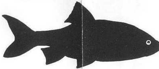
Roach Rutilus Rutilus
